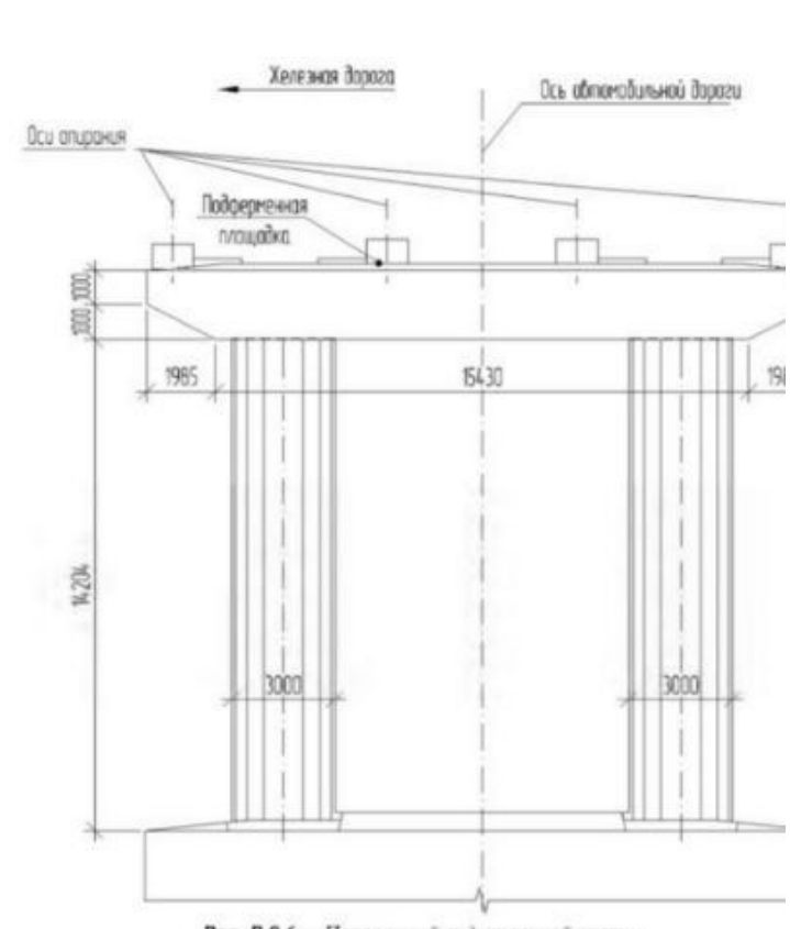
Рис. В.9.6 – Поперечный вид стоечной опоры
